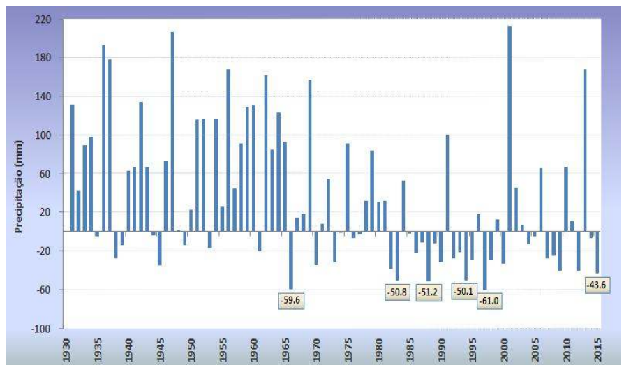
Figura 1 – Desvios da precipitação no mês de março em Portugal Continental (1931-2015)
