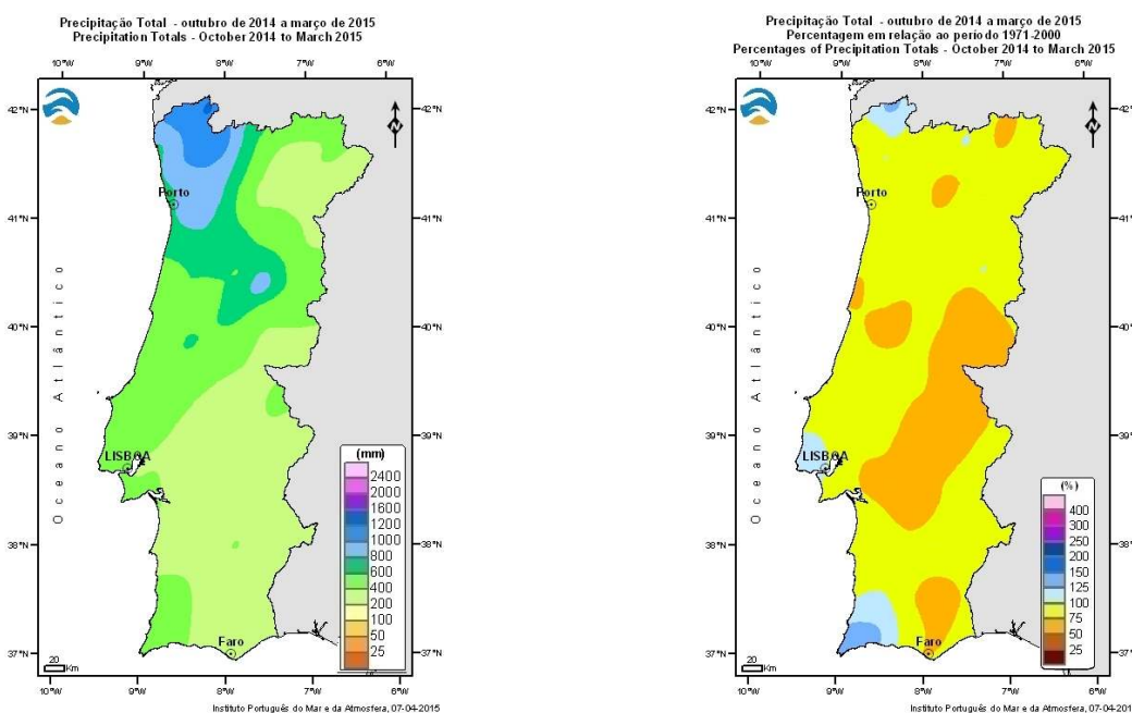
Figura 4 - Precipitação acumulada desde 1 de outubro 2014 (esq.) e percentagem em relação à média 1971-2000 (dir.)
