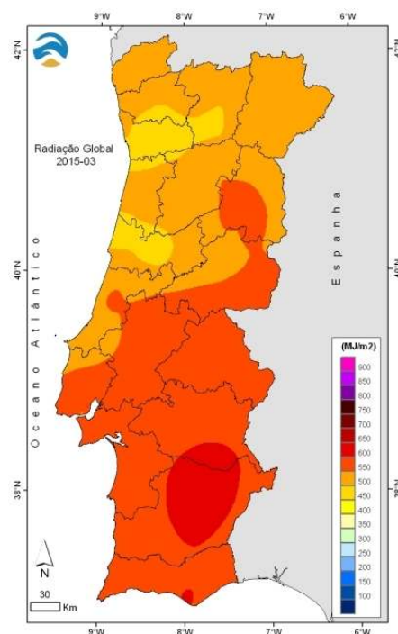
Figura 6 – Distribuição espacial dos valores da radiação solar global mensal ( \text{MJ/m}^2 ) em março de 2015
