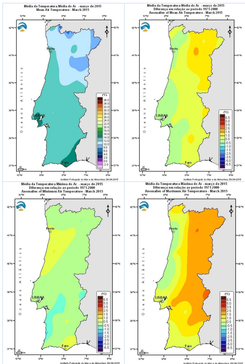
Figura 2 - Distribuição espacial dos valores médios da temperatura média do ar e anomalias da temperatura média, mínima e máxima do ar (em relação ao período 1971-2000), no mês de março de 2015.
